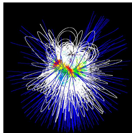
Carte du champ magnétique de SU Aurigae, une bébé-étoile située à environ 450 années-lumière du Soleil, scrutée en continu, à la fois par NARVAL et ESPaDOnS
